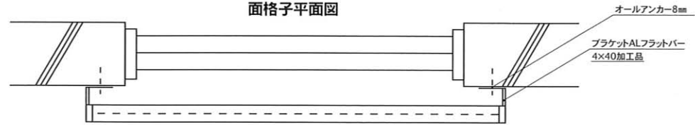
面格子平面図
